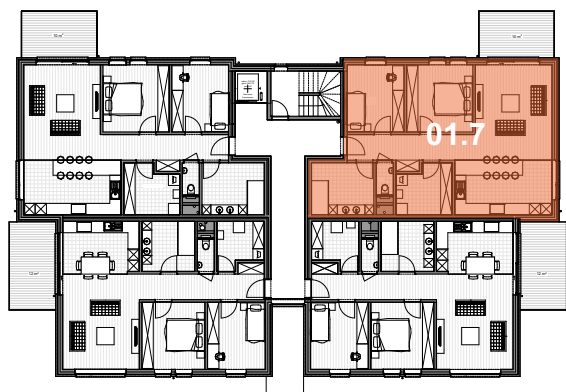
Plan général
